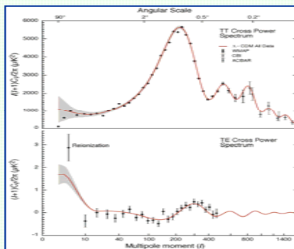
CMB (+ SN, H_0 , etc.)
