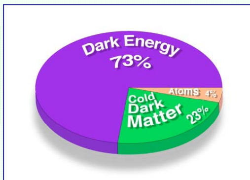
CMB (+ SN, H_0 , etc.)
